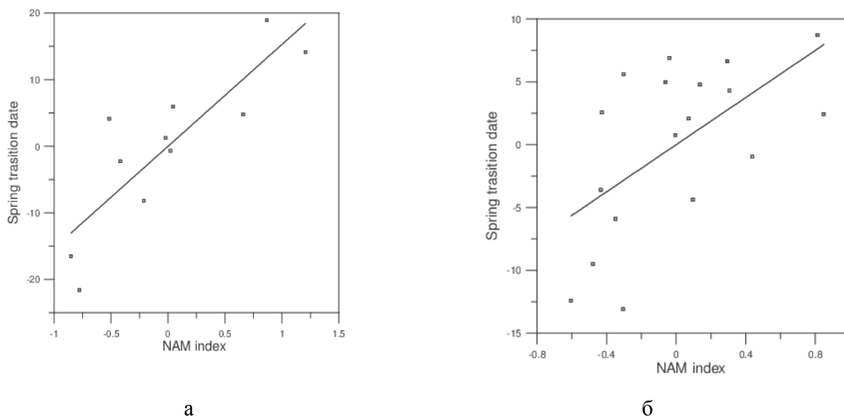
Рисунок 5 – Диаграмма рассеяния для ряда СКМ-индексов на уровне 10 гПа, осредненных за март – апрель, и временного ряда ранних дат весенней перестройки в случае восточной фазы КДК в марте (а) и временного ряда дат ранней весенней перестройки (б)
