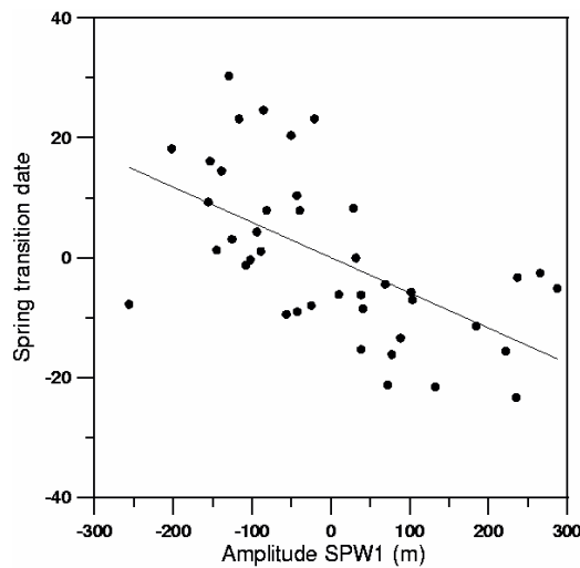
Рисунок 3 – Диаграмма рассеяния между амплитудами СПВ1 на уровне 30 гПа и датами весенней перестройки на уровне 10 гПа, рассчитанными по данным NCEP/NCAR
