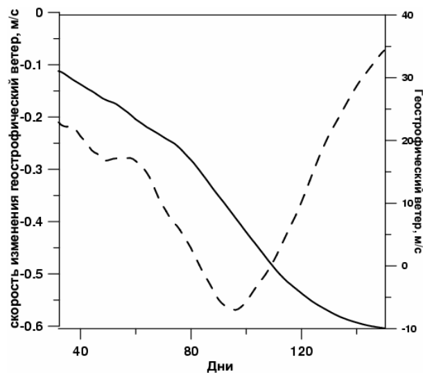
Рисунок 1 – Климатическое изменение зональной компоненты скорости геострофического ветра (сплошная линия) и сглаженная скорость ее изменения в февралемарте (штриховая линия), рассчитанные по данным UK Met Office, на уровне 10 гПа, 67.5°N
