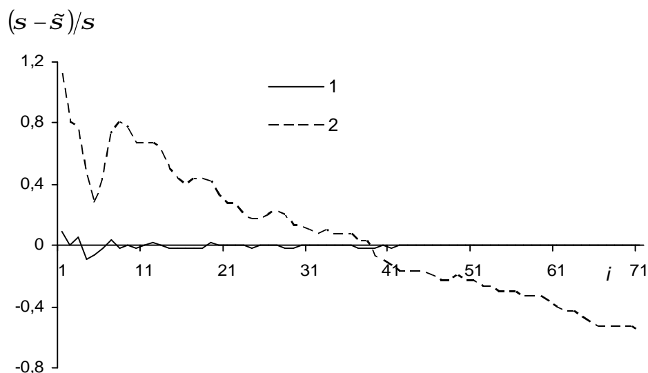
Рис.4. Зависимость величины \delta\sigma/\sigma , найденной путем решения прямой и обратной задачи от числа шагов
