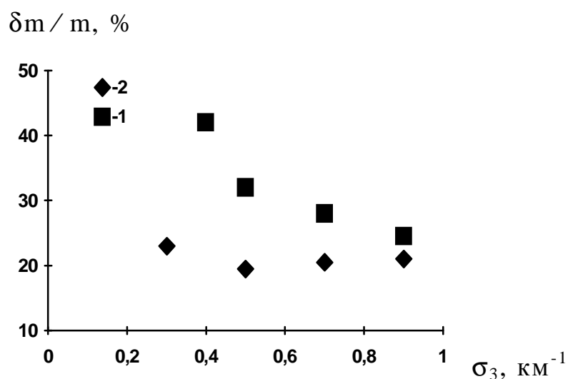
Рис.2. Точностные характеристики треугольной схемы, углы зондирования 90^\circ, 30^\circ, m=1 , 1 - \sigma_3/\sigma_2 = 0,5 ; 2 - \sigma_2 = 2 \text{ км}^{-1}
