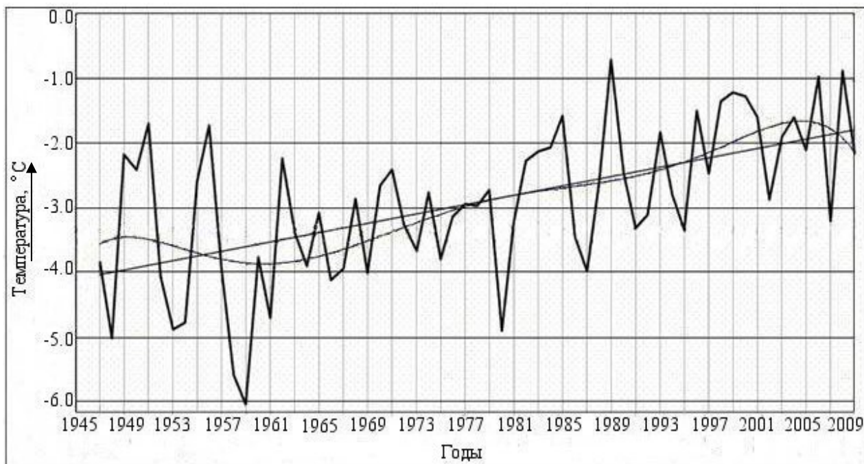
Рисунок 1 – Изменение среднегодовых аномалий температуры воздуха в регионе Антарктического полуострова (с 1947 по 2009 гг.)
