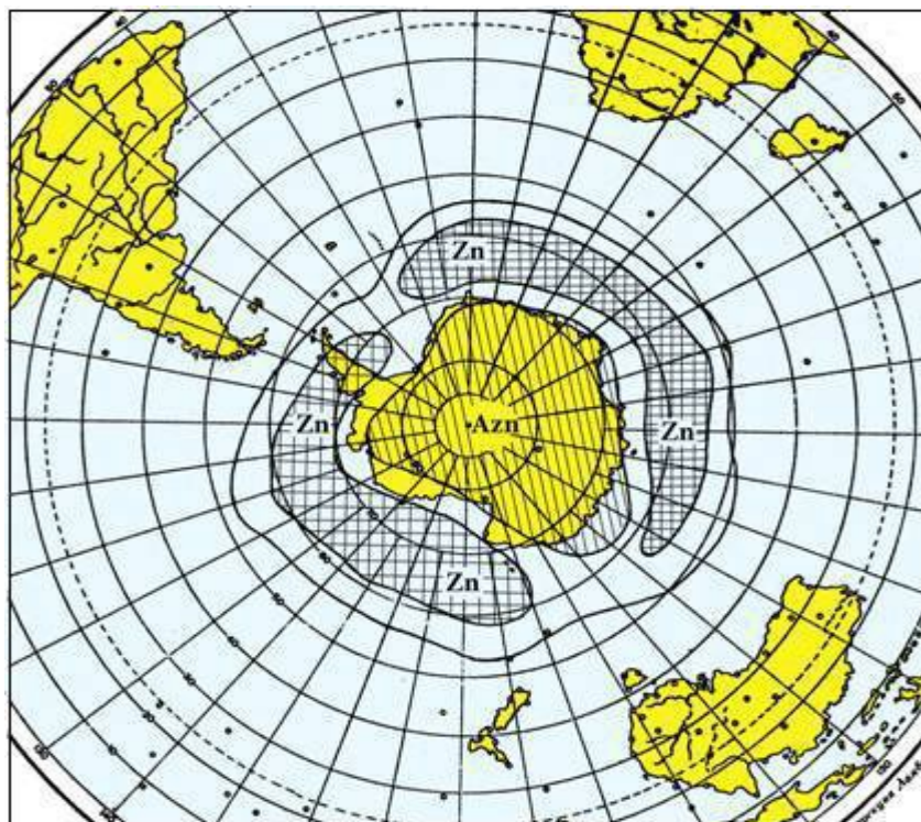
Рисунок 5 – Расположение приземных центров барических образований над Южной полярной областью в экстремально теплые годы
