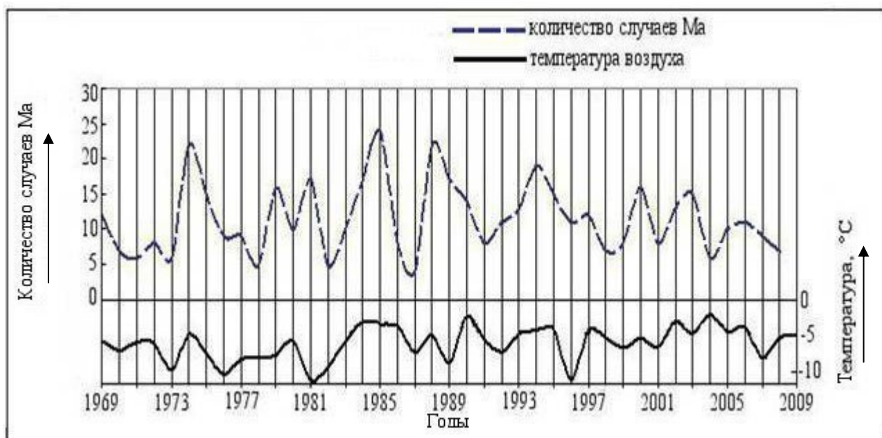
Рисунок 3 – Количество случаев (число дней) формы Ма циркуляции атмосферы и многолетний ход температуры воздуха на ст. Беллинсгаузен для августа месяца
