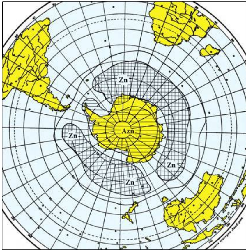
Рисунок 4 – Расположение приземных центров барических образований над Южной полярной областью в экстремально холодные годы
