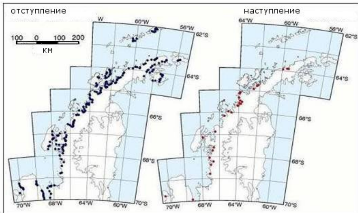
Рисунок 2 – Общее изменение фронтов ледников на Антарктическом полуострове (отступление/наступление) с 1954 года
