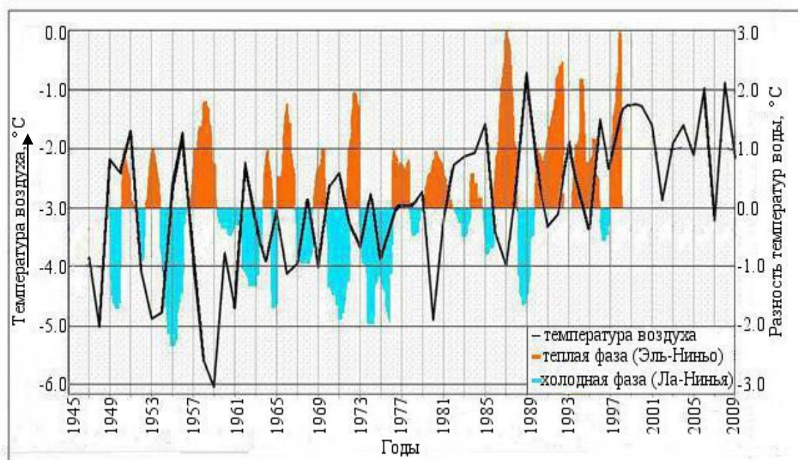
Рисунок 6 – Среднегодовые аномалии температуры воздуха в регионе Антарктического полуострова и фазы явления Южной осцилляции (разность температур воды)
