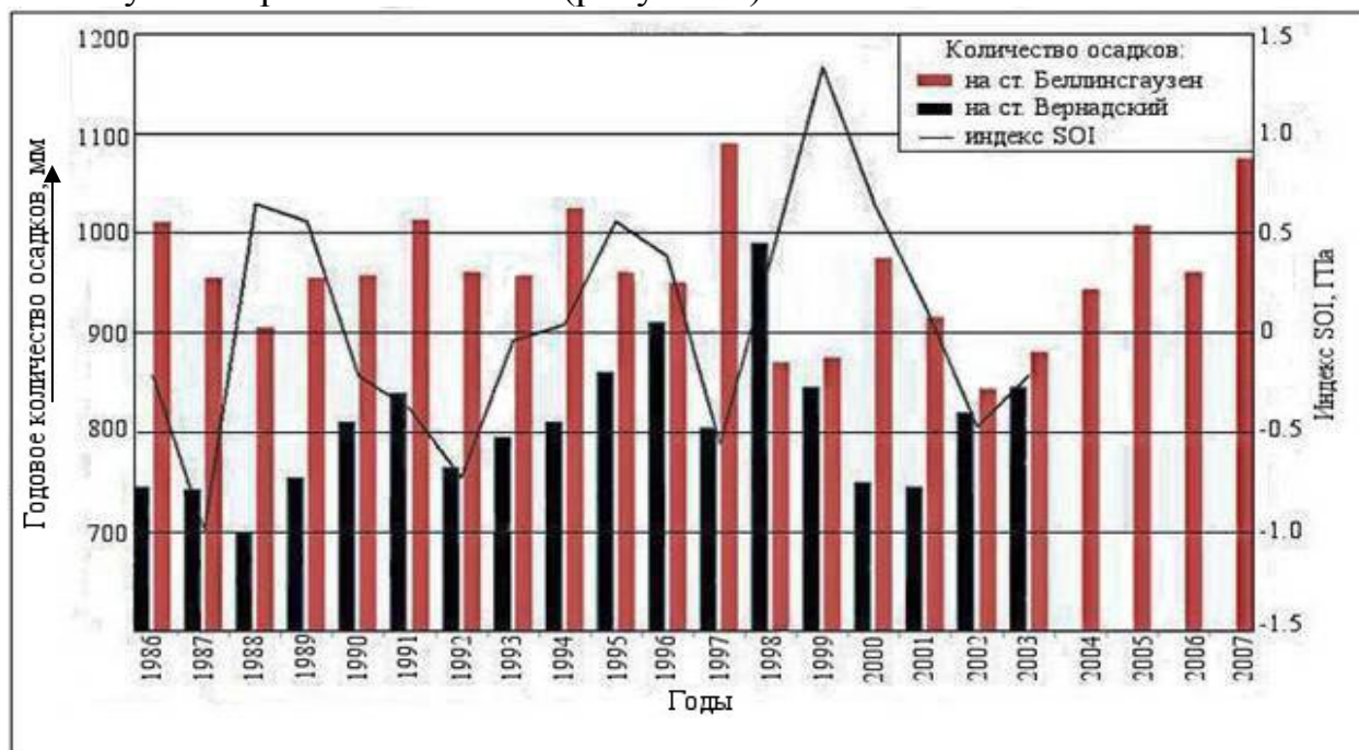
Рисунок 7 – Годовое количество осадков на станциях Беллинсгаузен и Вернадский и индекс Южной осцилляции (SOI)
