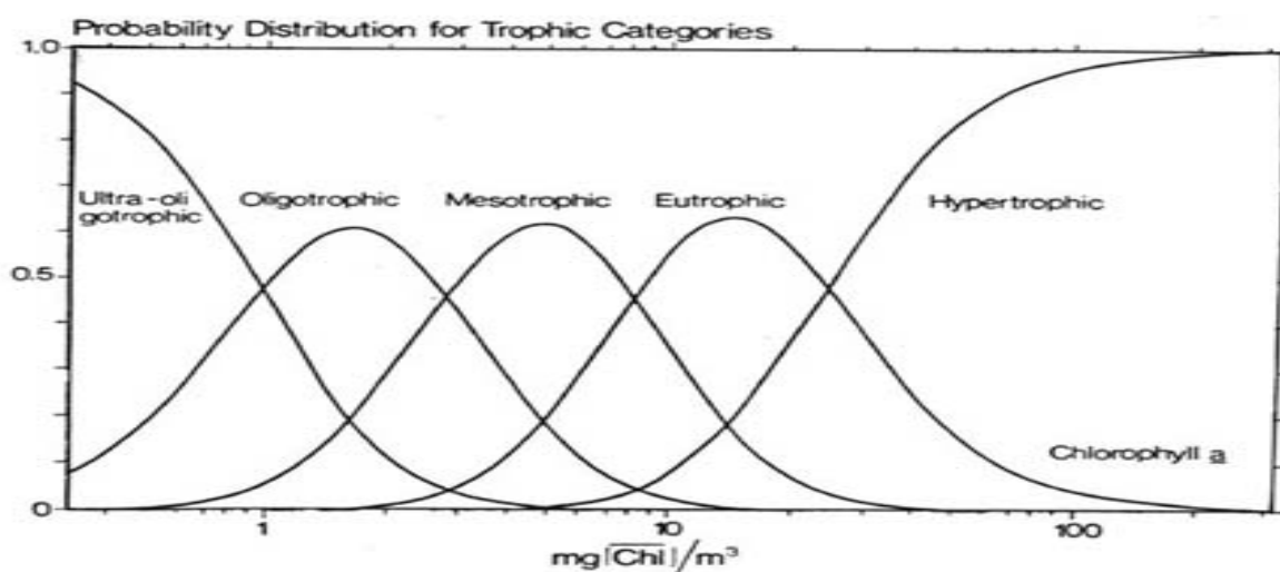
Рисунок 2 - Вероятностная классификация для установления трофического статуса по содержанию хлорофилла «a»
