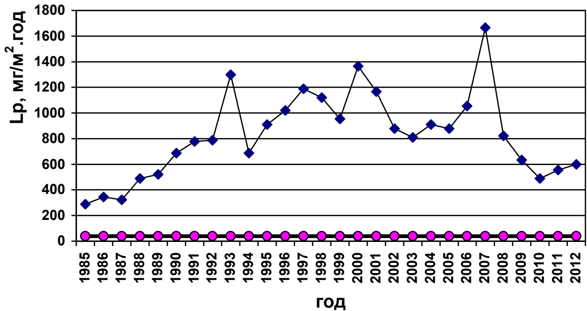
Рисунок 6 - Межгодовая динамика нагрузки фосфором общим на озеро Тайху (линия, параллельная оси абсцисс, – предельно допустимая нагрузка)
